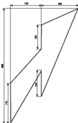
Planche 10. Ilots directionnels.
